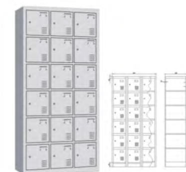
JF-3B6A H1850 × W900 × D400mm
